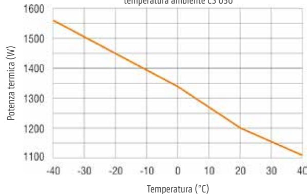
Diagramma della potenza termica in funzione della temperatura ambiente CS 030
