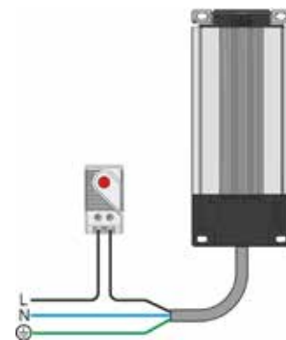
Esempio di collegamento
