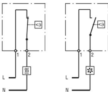
Termostato STO 011 (NC) Termostato STS 011 (NO)
