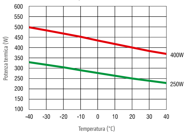
Diagramma della potenza termica in funzione della temperatura ambiente CSF 028
