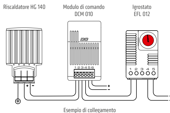
Esempio di collegamento
