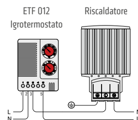
Esempio di collegamento
