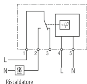
Schema di collegamento
