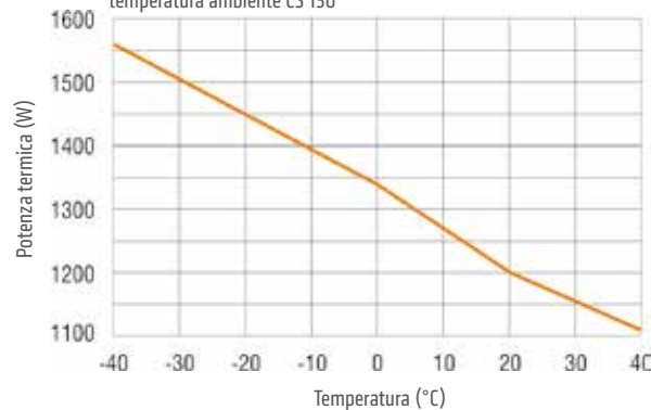
Diagramma della potenza termica in funzione della temperatura ambiente CS 130
