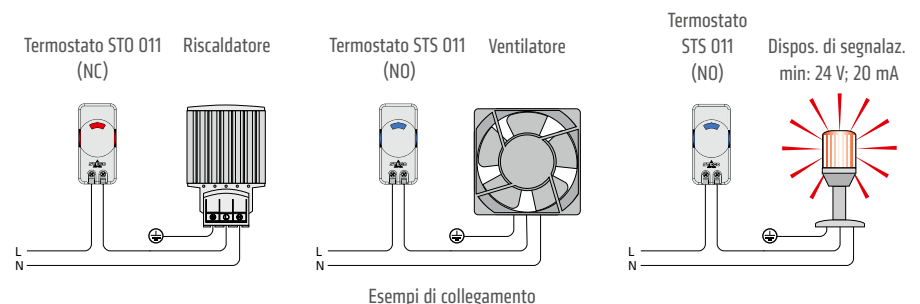
Esempi di collegamento
