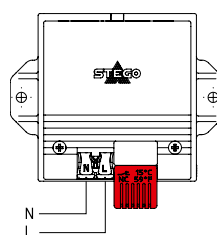
Esempio di collegamento Ventilatore di riscaldamento CSF 028
