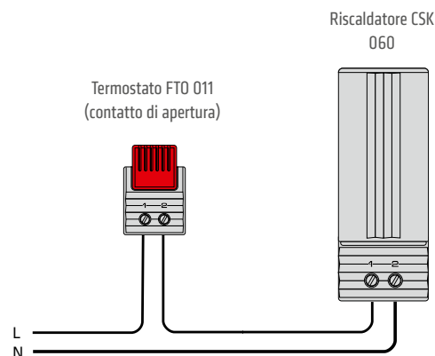
Esempio di collegamento
