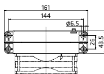
Fissaggio a vite
