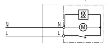
Schema di collegamento
