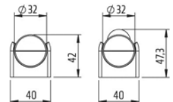
Vista di lato della versione con fissaggio con clip
