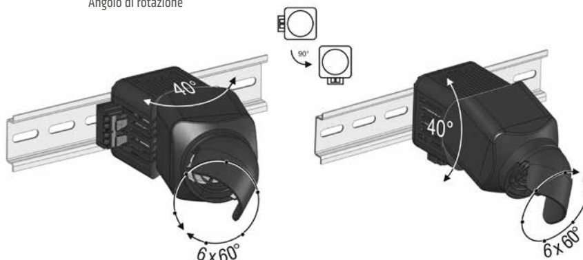
Angolo di rotazione
