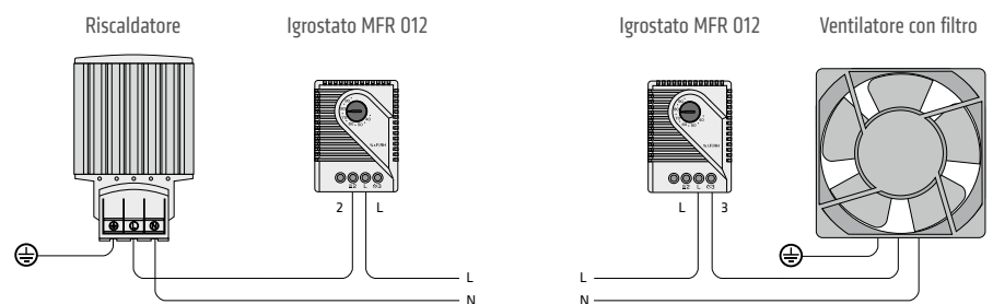
Esempi di collegamento
