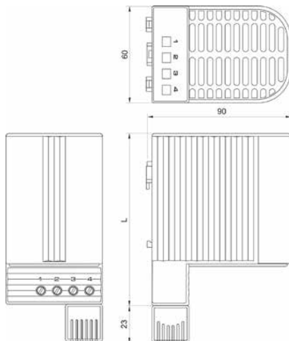
Riscaldatore CSF 060 50 W
